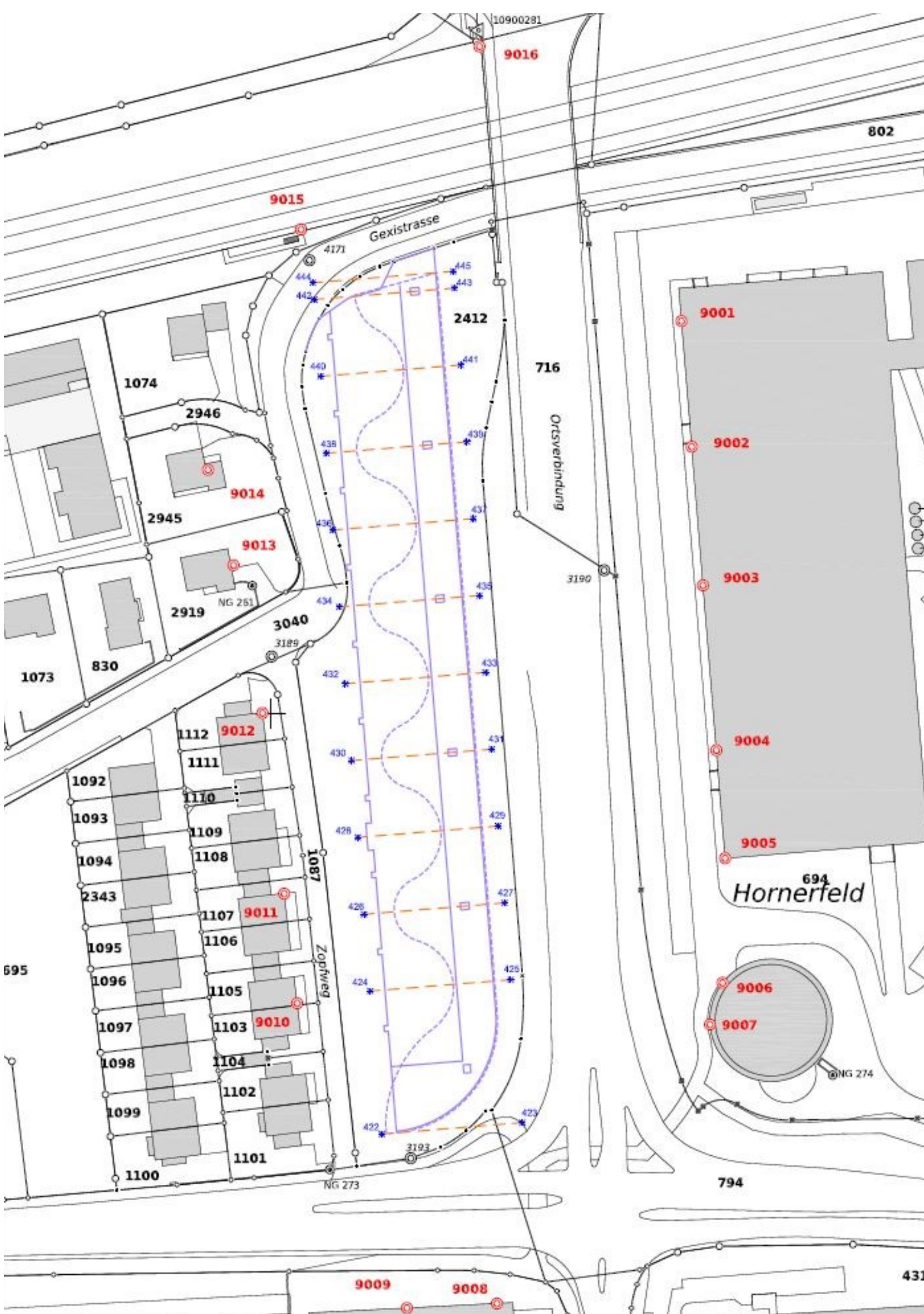
Übersichtsplan Baufixpunkte
