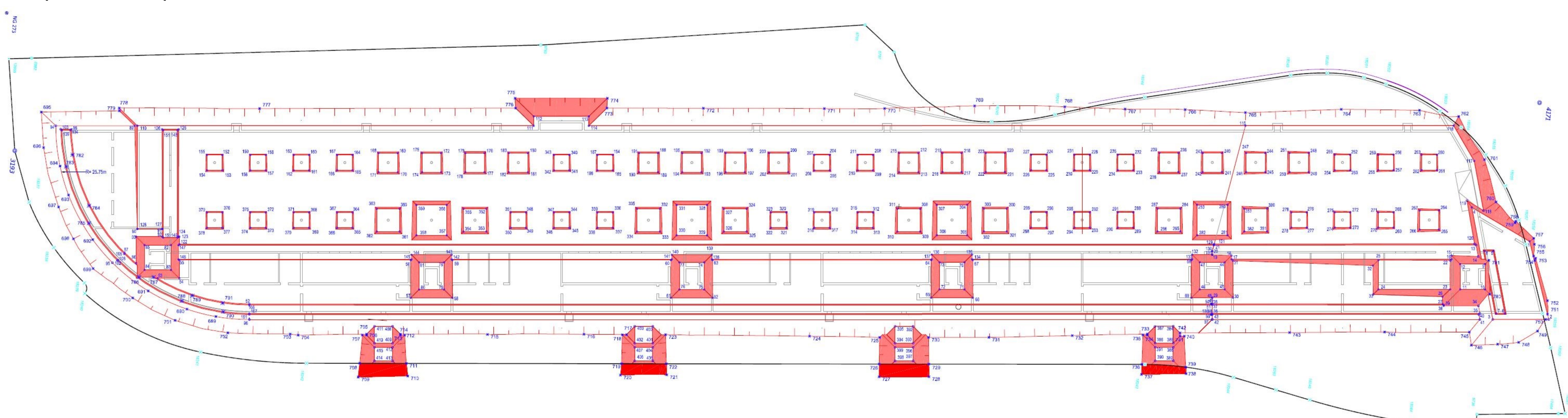
Aushubplan mit Bruchkanten und Punkten welche in einer separaten Koordinatenliste abgegeben wurden
